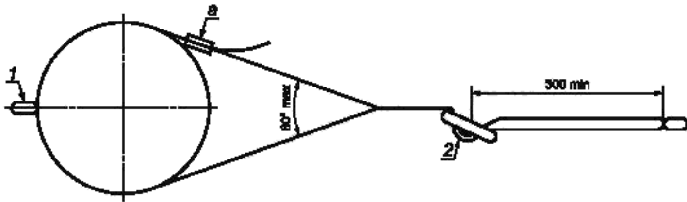
1 — соединительный элемент; 2 — регулятор длины A — пряжка, которая не должна находиться в контакте с цилиндром
